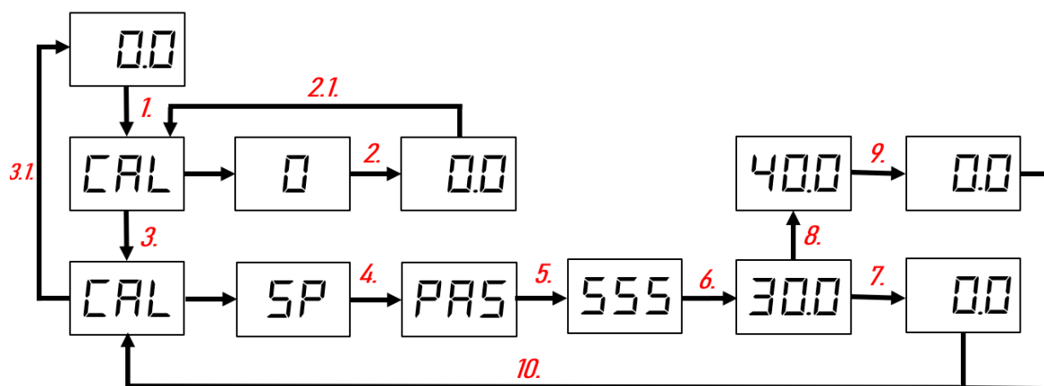
Рисунок 5 - Меню калибровки GS-02
