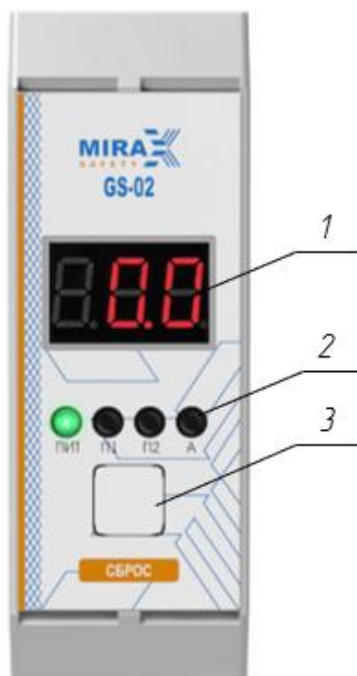
Рисунок 3 – Лицевая панель GS-02-I-D
